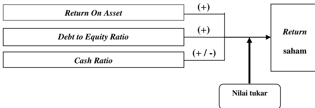
Gambar 2 Kerangka Pemikiran
