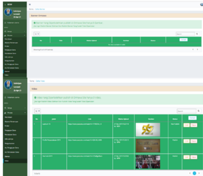
Gambar 9. Fitur Tambahan
