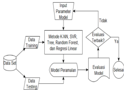
Gambar 1. Siklus eksperimen model
