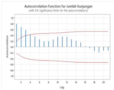
Gambar 3. Grafik ACF jumlah kunjungan
